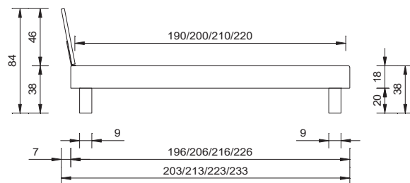
Seitenansicht vue de côté
